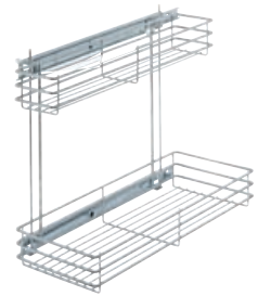
3 Unterspülen-Auszug für Küchenschwämme und Putzmittel
