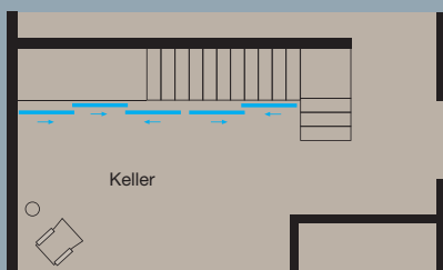
Maßgenau eingepasste schräge Türflügel füllen den Bereich unter der Treppe millimetergenau.
